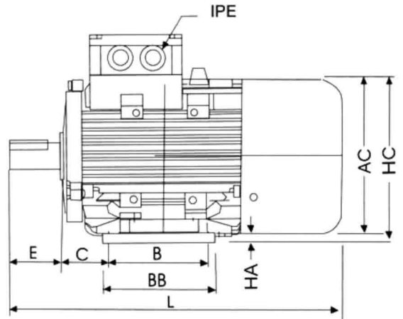
Tvar IMB3
