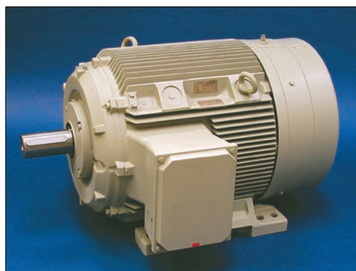
Motory tvaru IM B3 velikostí 180M až 315L Skříň svorkovnice na pravé straně
