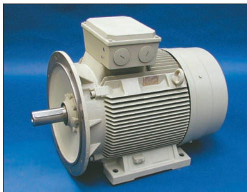
Motory tvaru IM B35 velikostí 180M až 315L Standardní provedení
